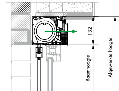
Opbouw Fixscreen® Mono AK EVO - Small
