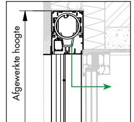
Voorbouw, geïntegreerd met kast in pleisterwerk
