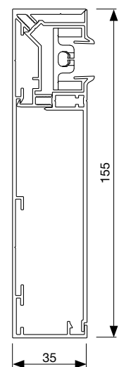
Diepe zijgeleider (D)
