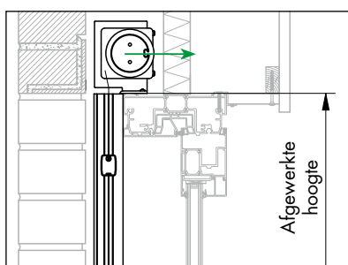
Inbouw, met beugels, zonder kast
