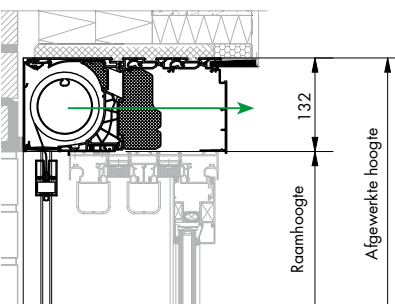
Opbouw Fixscreen® Mono AK EVO - XX-Large
