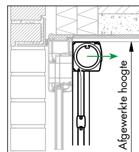
Voorbouw, voor het raam binnen
