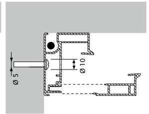
Zijdelingse montage zijgeleider Fixscreen® 100 EVO
