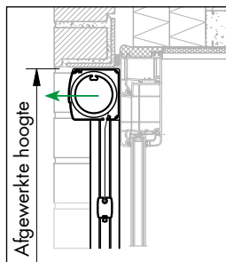
Voorbouw, voor het raam buiten
