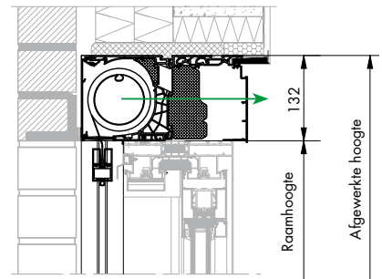
Opbouw Fixscreen® Mono AK EVO - X-Large
