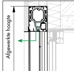
Voorbouw, geïntegreerd met kast in pleisterwerk
