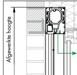
Voorbouw, geïntegreerd met kast
