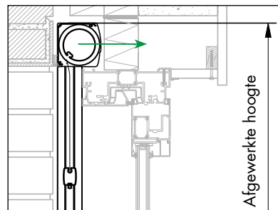
Opbouw, bovenop het raam met omgekeerde kast, zonder voorkap
