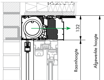
Opbouw Fixscreen® Mono AK EVO - Large
