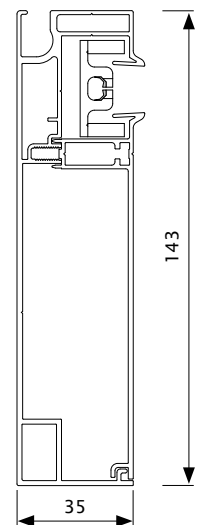
Diepe zijgeleider (D)
