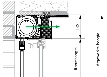
Opbouw Fixscreen® Mono AK EVO - Medium
