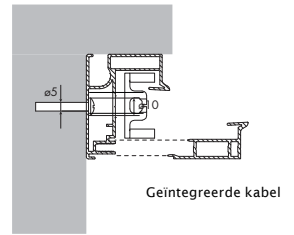
Zijdelingse montage zijgeleider Fixscreen® 150 EVO (F)
